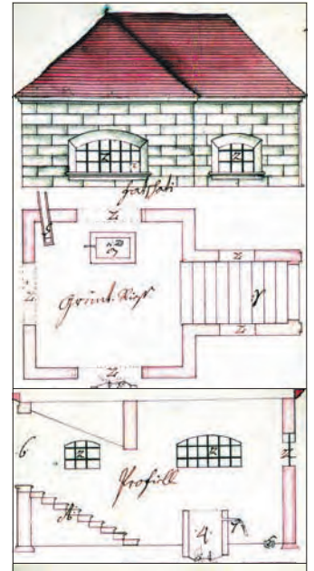
Fassade, Grund- und Aufriss zum Brunnenhaus in Großalbershof, kolorierte Federzeichnung von 1770.
